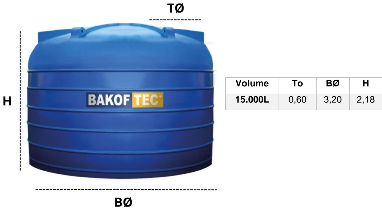
Figura 01. Desenho Tanque 15.000L Bakof Tec*.
